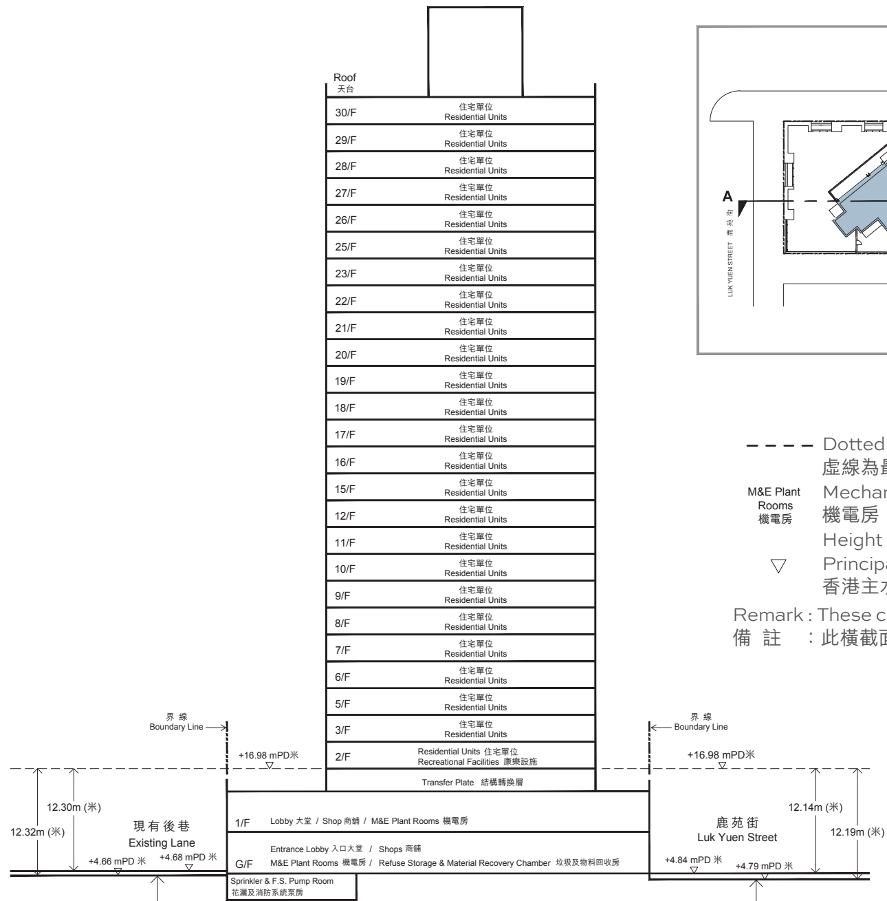
Cross-Section A-A 橫截面圖 A-A
